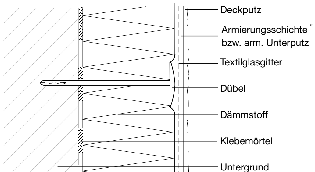
Schematischer Systemaufbau
